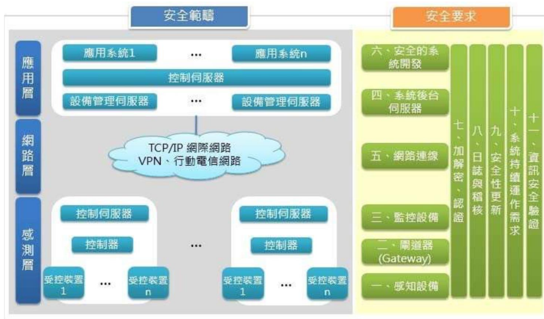
圖19、民生公共物聯網資訊安全領域
