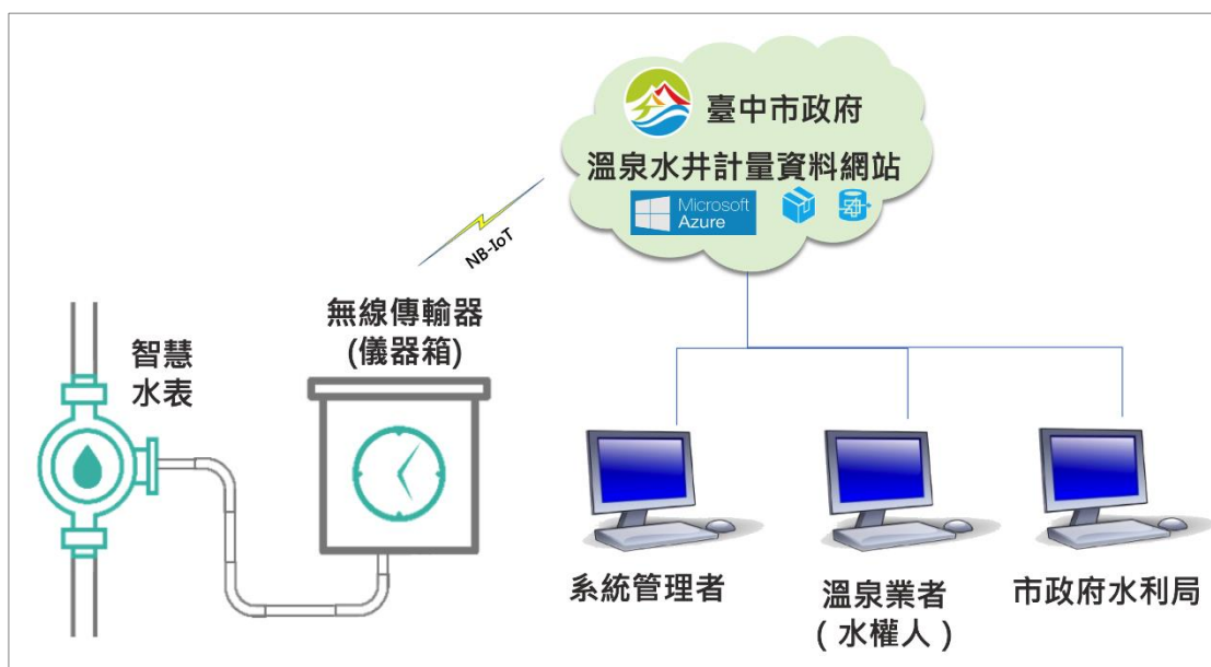
圖6、水井計量設備與資料傳輸應用架構圖
