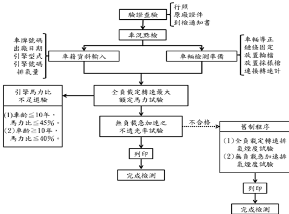
柴油車排煙檢測流程
