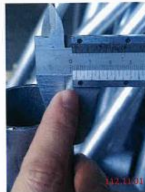
照片 3(抽測燈桿與燈具轉接桿，桿件長邊之管徑厚度 3mm，尚符契約規範)
