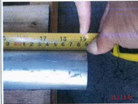
照片 1(抽測燈桿與燈具轉接桿，桿件長邊之長度 48.6cm，尚符契約規範)
